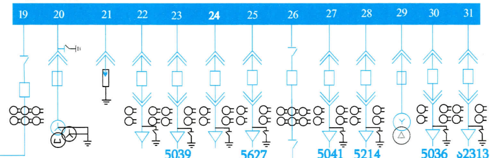
6 კვ II სექცია
