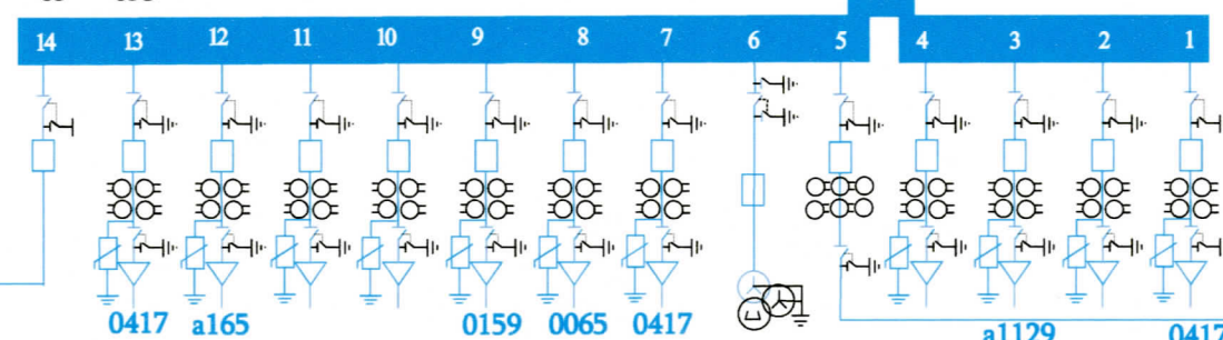
გგ III სექცია
