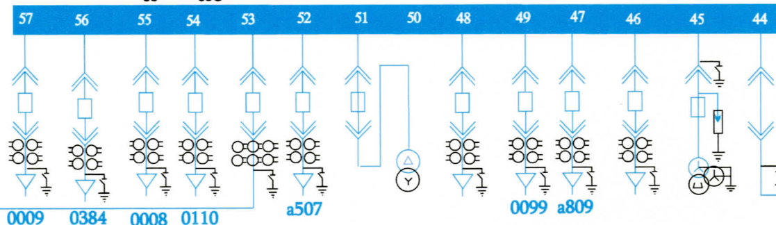
გგ IV სექცია
