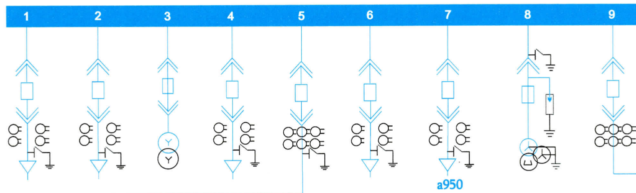
6კვ. I სექცია
