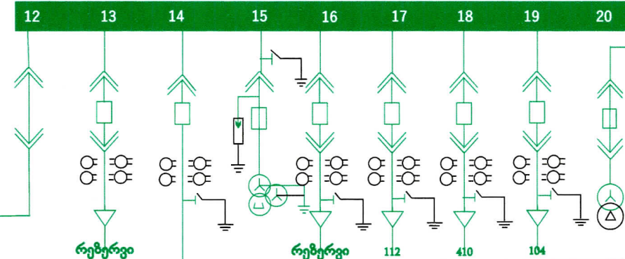
10 კვ II სექცია
