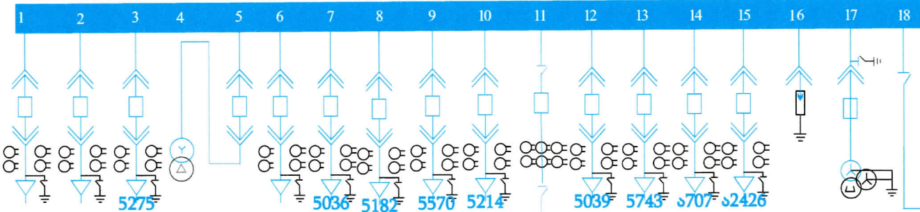
6 კვ I სექცია
