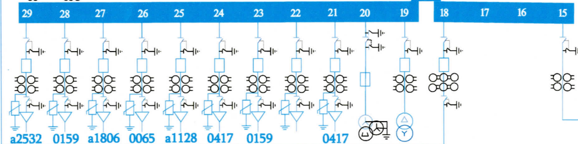
გგ II სექცია
