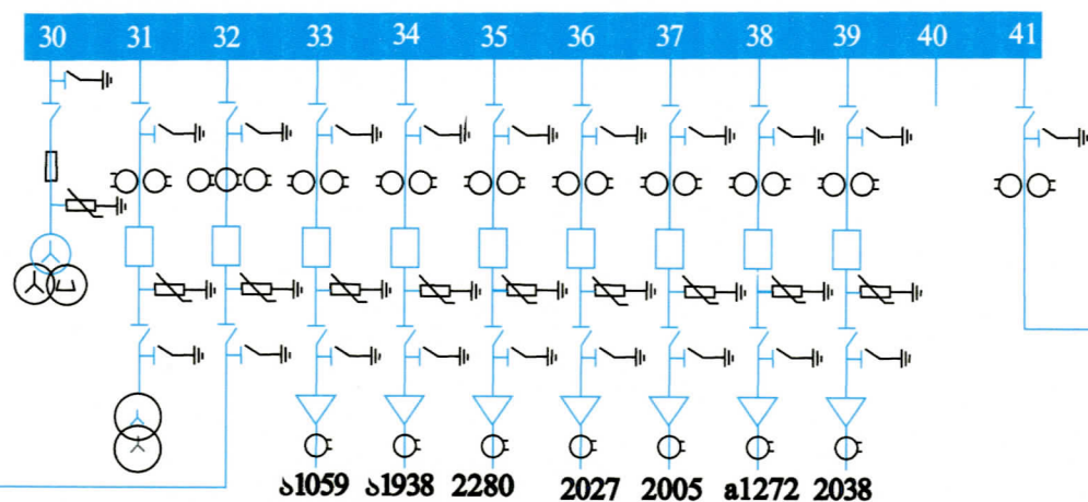
6კვ III სექცია
