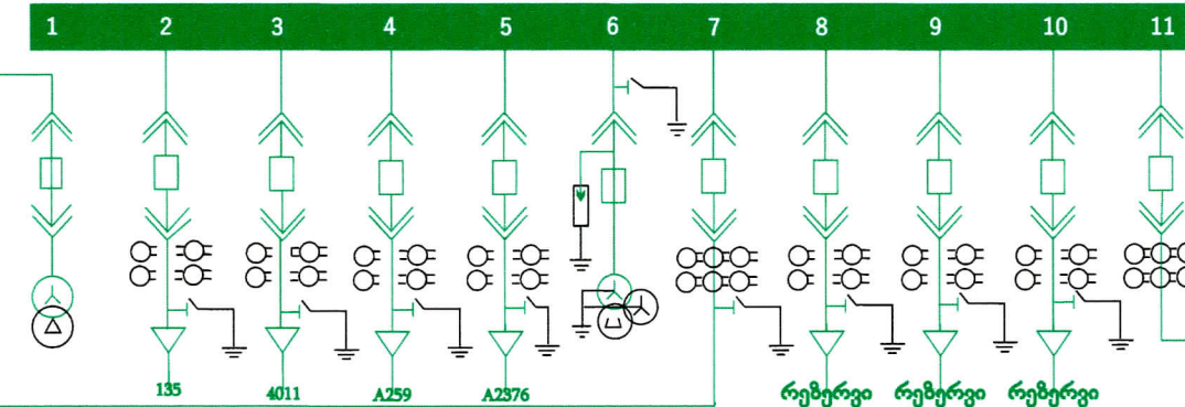
10 კვ I სექცია
