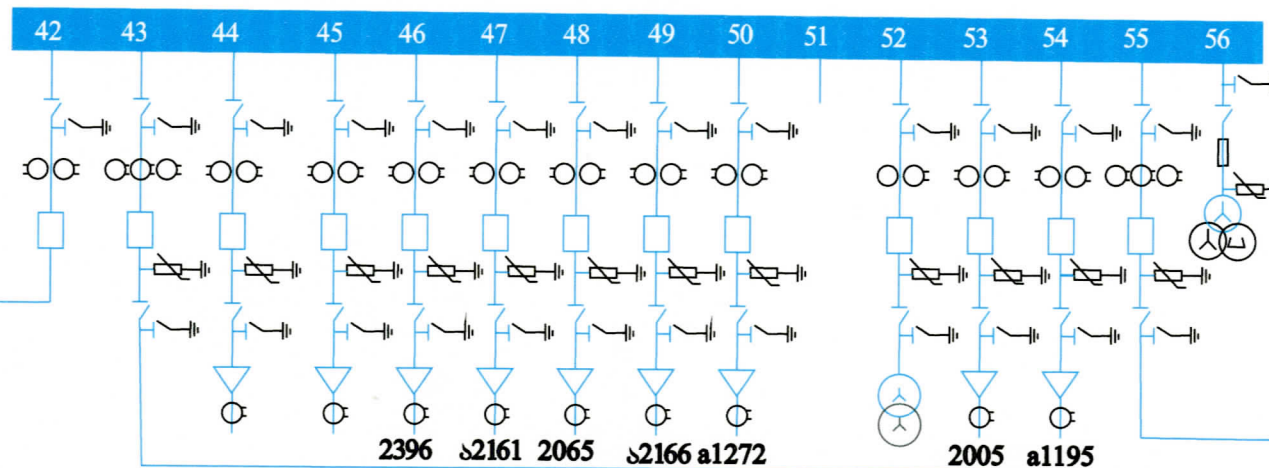
6კვ IV სექცია
