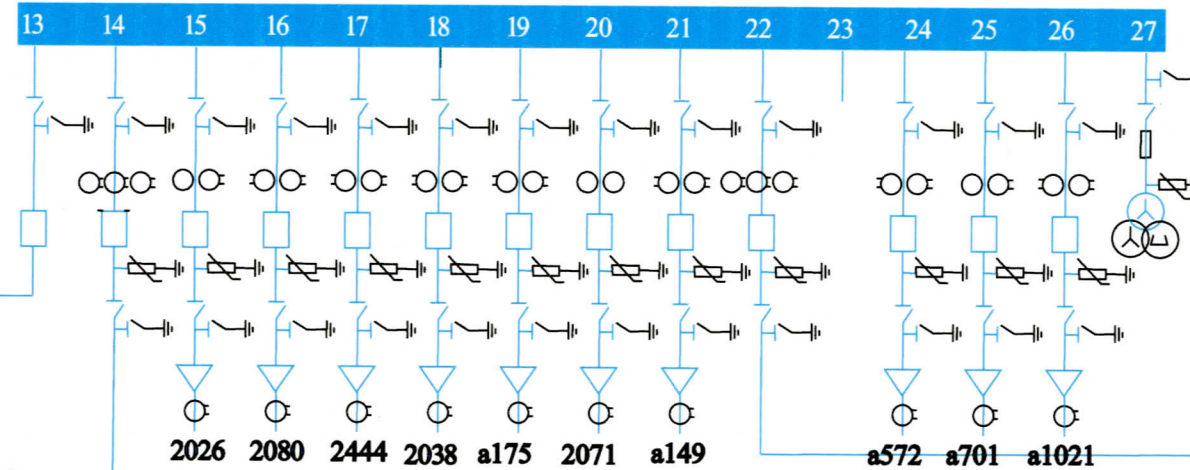
6კვ II სექცია
