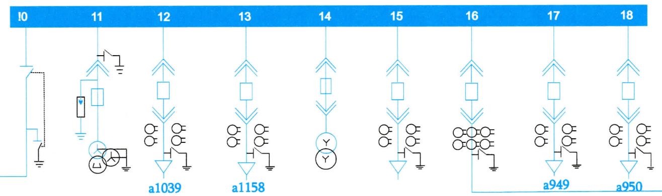
6კვ. II სექცია
